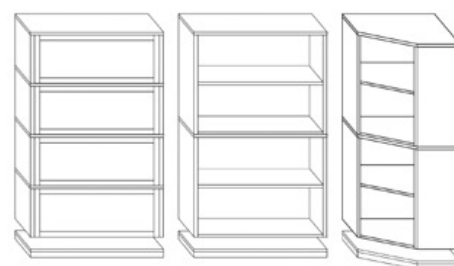
Korpuselemente 28, Höhe je Element 339/678 mm, Tiefe 280 mm.
