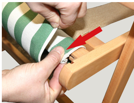
Schritt 3 Ziehen Sie nun die Stofflasche über die gesamte Breite aus der Nut heraus, um die Bespannung zu lösen.
